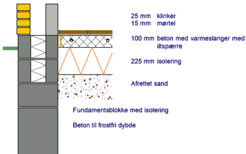
Figur 8. Gulvarme i betongulv med fundamentsblokke med isolering.
