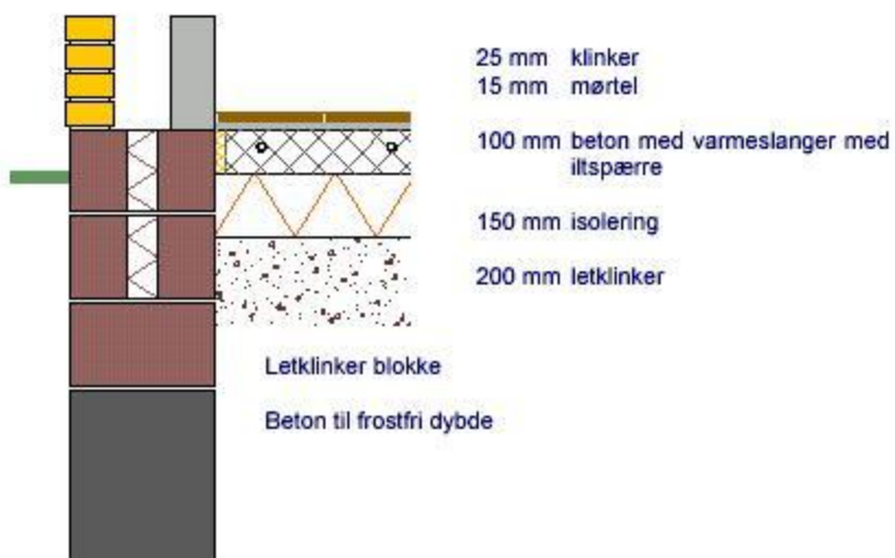
Figur 9. Gulvarme i betongulv med letklinkerblokke.
