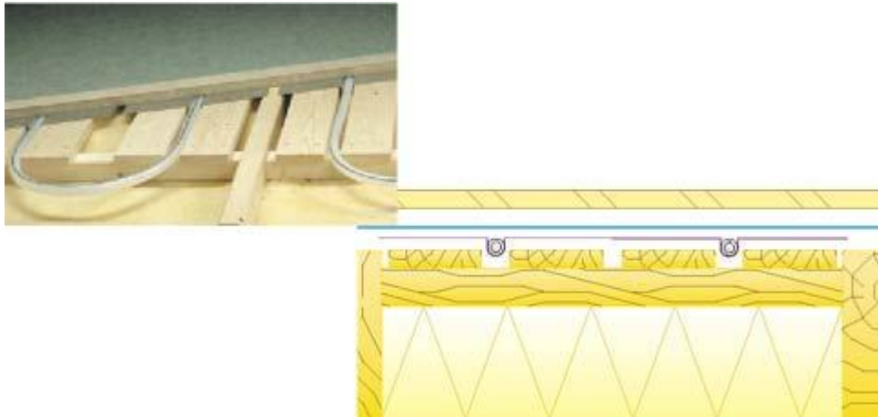
Figur 10. Gulvvarmeslanger med varmfordelingsplader nedlagt i bjælkelag. Det skal sikres, at bjælkerne har den fornødne styrke til at kunne klare udskæringerne. Kilde: Unopor Wirsbo A/S
